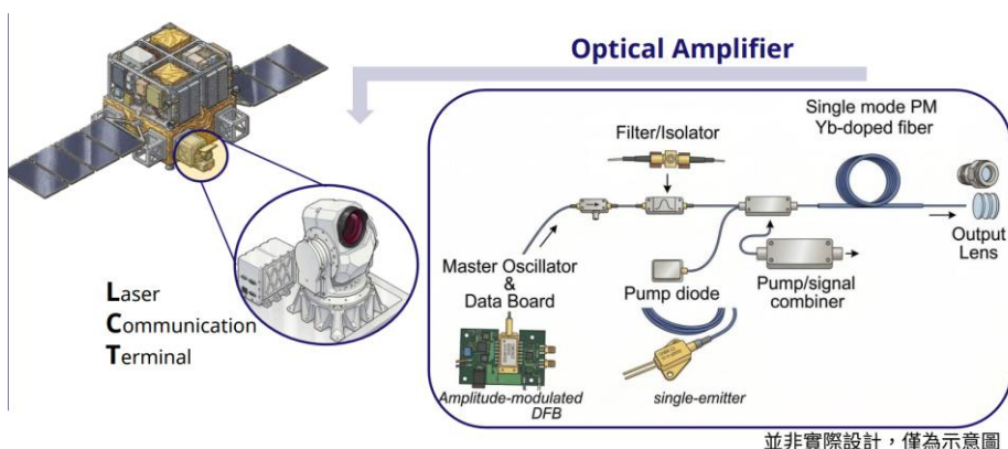
圖表六：衛星間光通訊元件示意圖
