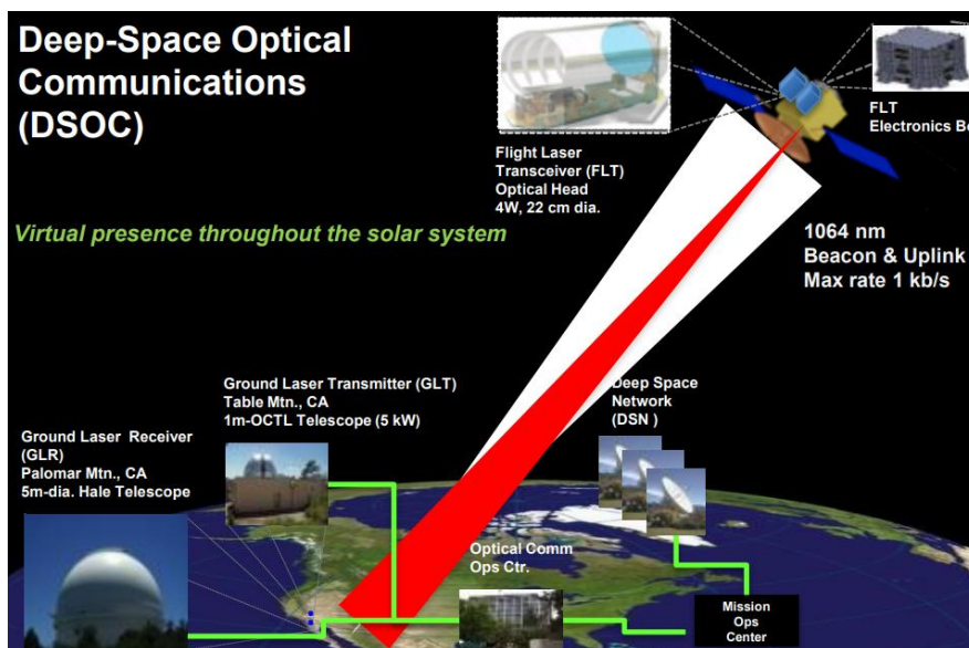
圖表八：衛星對地面雷射通訊
